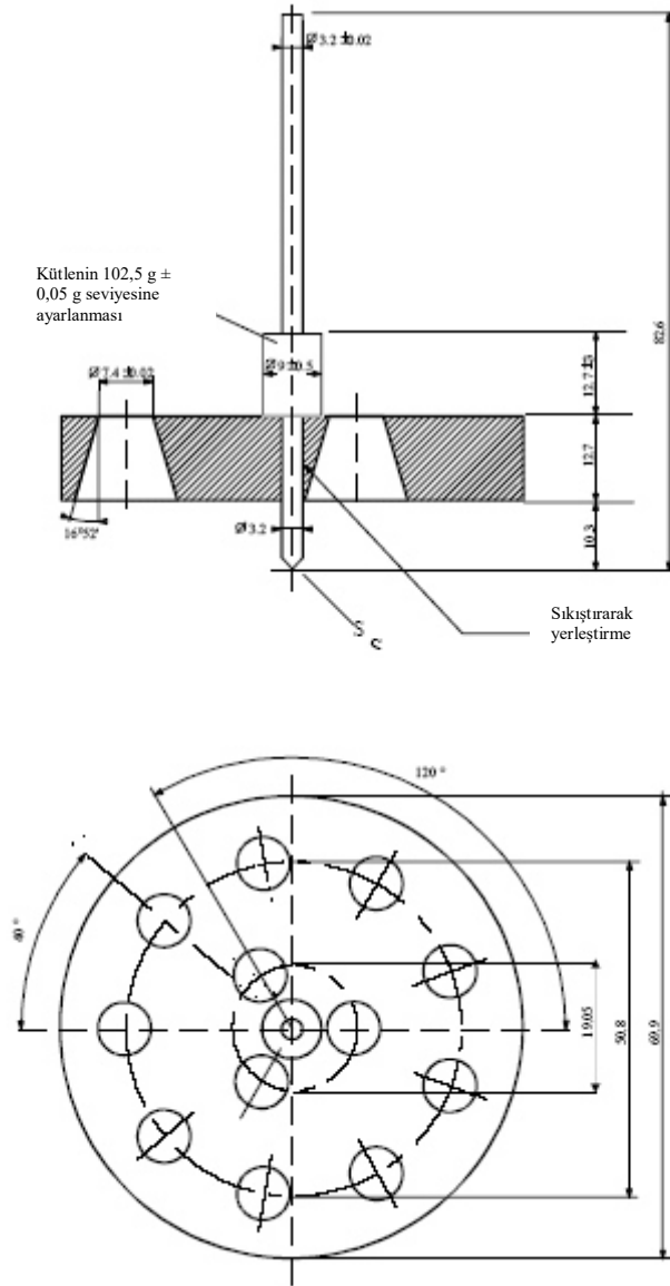
Şekil 1 - Penetrometre
